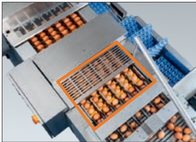
Kontinuierlicher Eierstrom: die Eier gelangen auf breiten Rollen in den Farmpacker → kein Kontakt der Eier untereinander und dadurch sicherer Weitertransport
