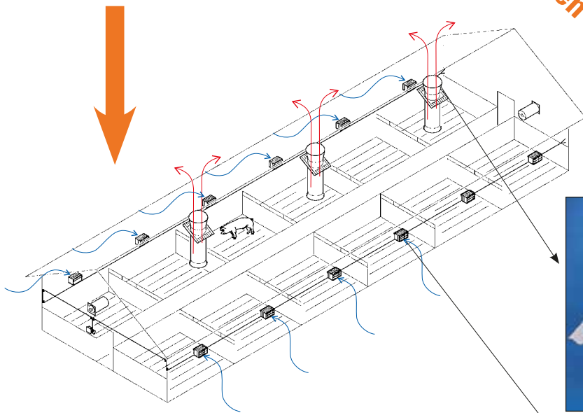
135pro – steuert das gesamte Stallklima
